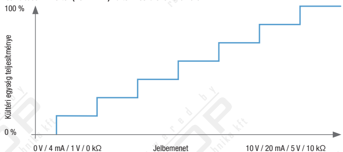
Teljesítmény-meghatározás 8 fokozatban Power Inverter (PUHZ-RP) és Zubadan Inverter (PUHZ-HRP) kültéri készülékek számára.
