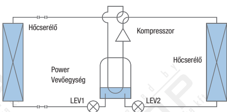
A Power Receiver és a 2 expansziós szelep maximális hatékonyságot biztosít.
